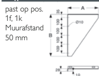
Zijplaten voor wandmontage*
