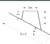
Dakdoorvoer 26° - 35°
