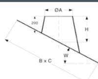
Dakdoorvoer 36° - 45°
