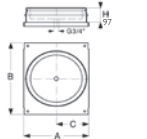
Zijplaten voor wandmontage*
