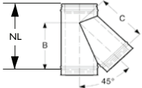
T-aansluitstuk 45°, met condensgroef
