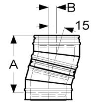
Afb. Bocht 30°
