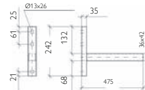
Verlengde muurconsole (paar)*
