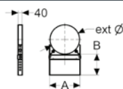
Muurbeugel (verstelbaar) 75-300 mm
