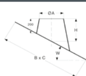
Dakdoorvoer 16° - 25°
