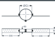
Daksteun
