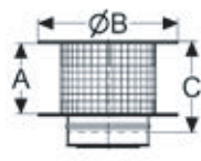
Regenkap Anti-Splash met draad + klemband
