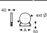
Lichte muurbeugel
