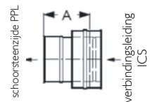
Aansluitingsovergang ICS naar PPL
