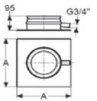
Grondplaat voor vloermontage, zijdelingse afvoer
